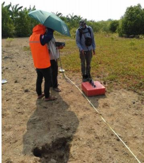
Gambar A.1 Akuisisi data GPR.
