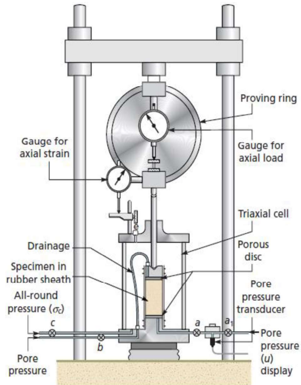
Gambar 3.11 Uji Triaksial [5]
