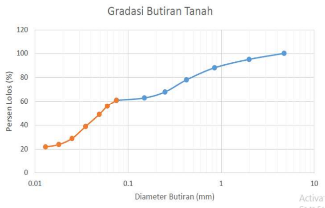
Gambar 3.7 Grafik gradasi butiran tanah [28]
