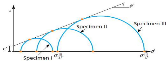
Gambar 3.12 Mohr circle pada uji triaksial CD [5]
