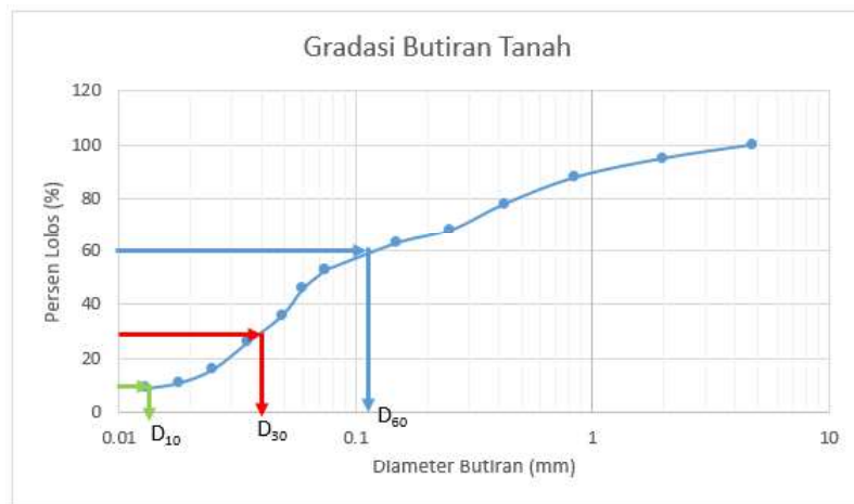
Gambar 3.9 Grafik gradiasi butiran tanah [28]
