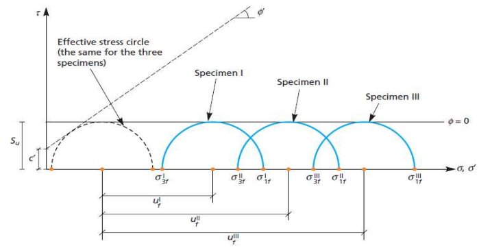
Gambar 3.13 Mohr circle pada uji triaksial UU [5]
